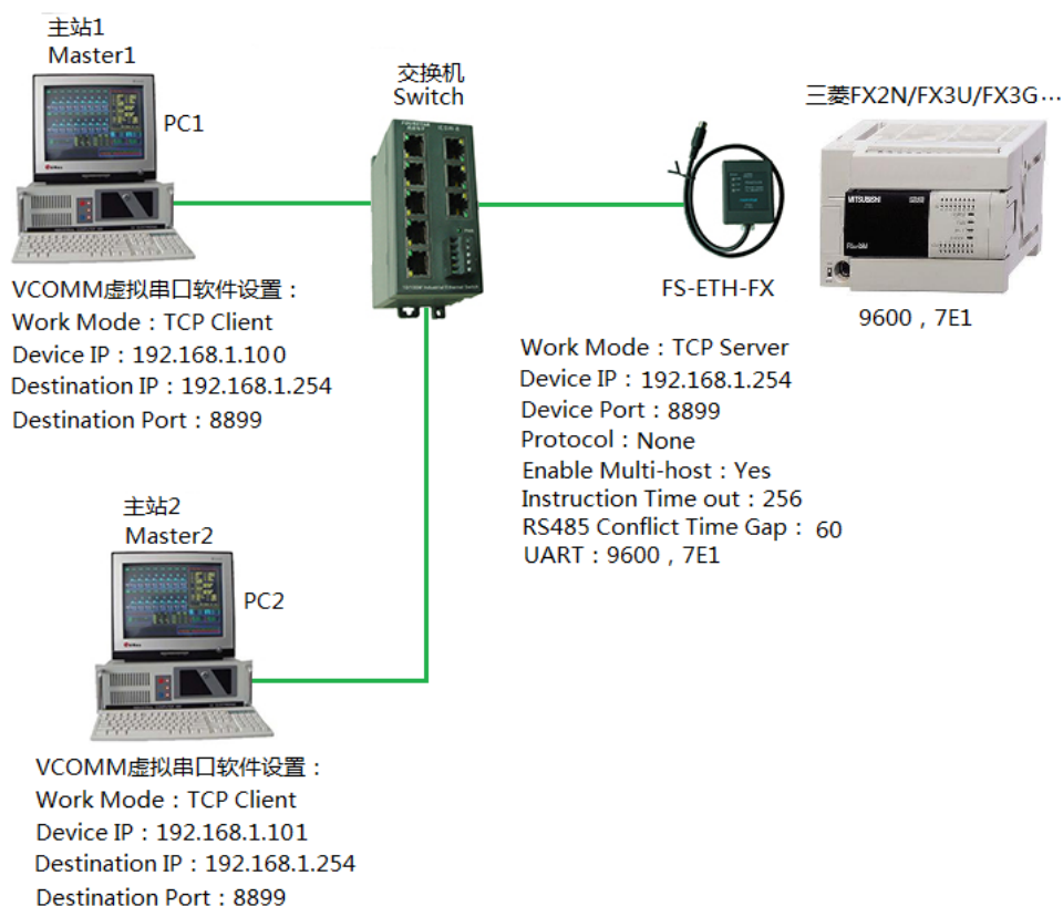
图 1-1 组态王与三菱 FX 系列 PLC 多主站通讯连接拓扑
