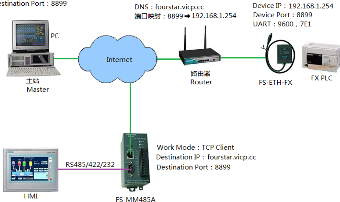
图5.3-1 FS-ETH-FX在互联网上的通讯网络拓扑
