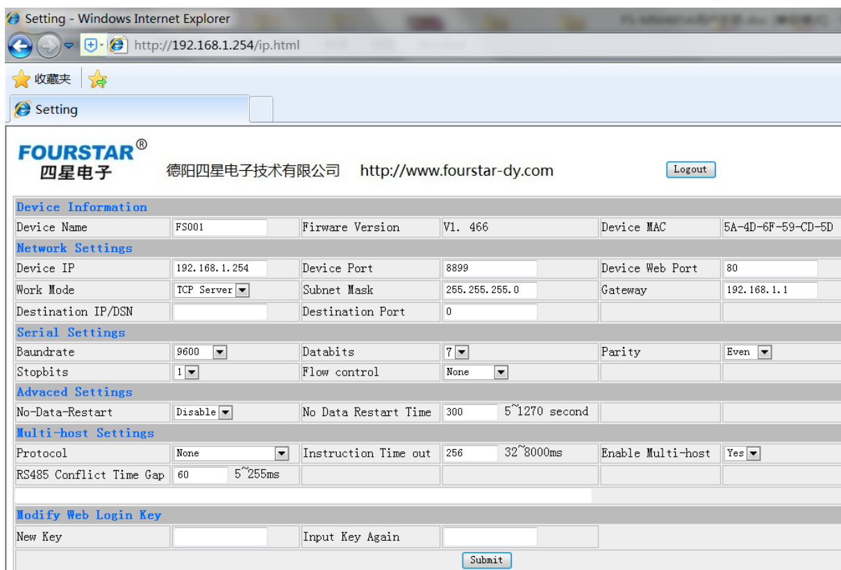
图5.2-1 FS-ETH-FX作多主站共享串口服务器时的设置
