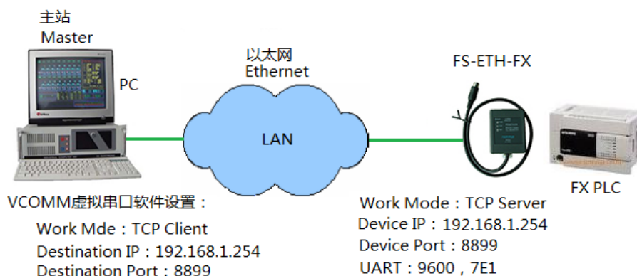
图5.1-1 计算机与FX系列PLC通过以太网通讯
