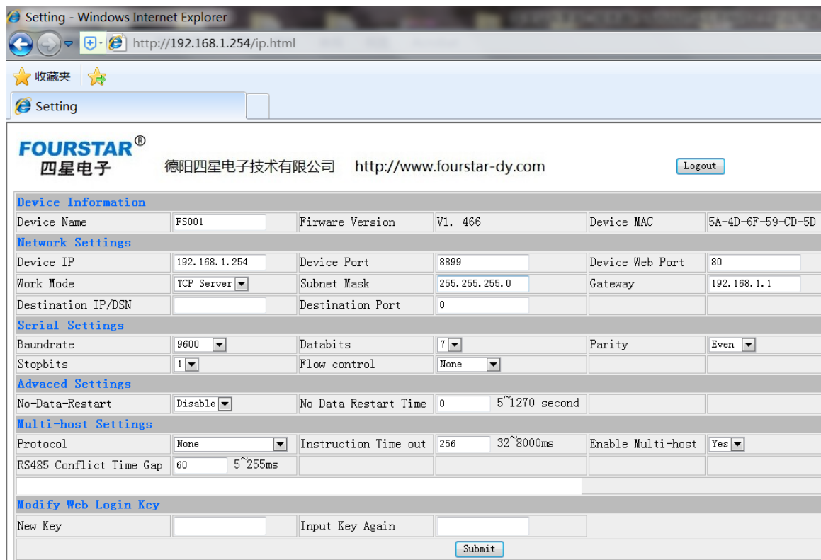
图 1-2 FS-ETH-FX 参数设置截图
