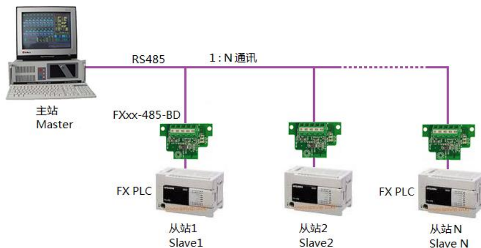
图 1-1 典型的单个主站 RS485 通讯网络拓扑
