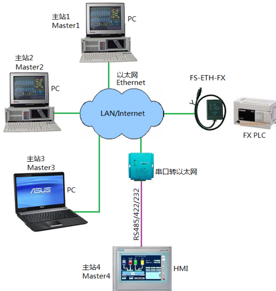
图 1-2 采用 FS-ETH-FX 的多主站通讯网络拓扑
